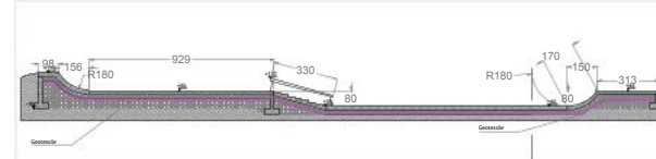
SEZIONI SPORTIVE PISTA SKATEBOARD scala 1:50
