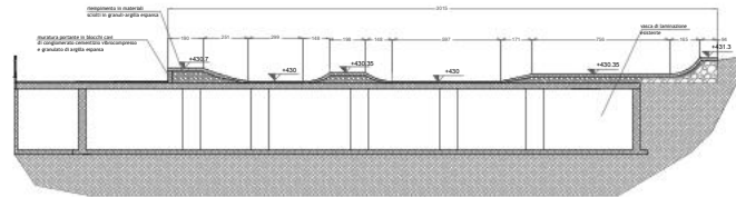
ASSONOMETRIA
