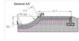
SEZIONI SPORTIVE PISTA SKATEBOARD scala 1:50
